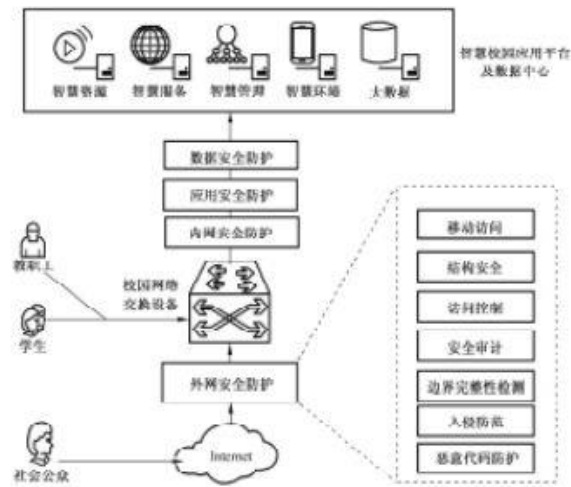
图 7 智慧校园信息安全防护架构
