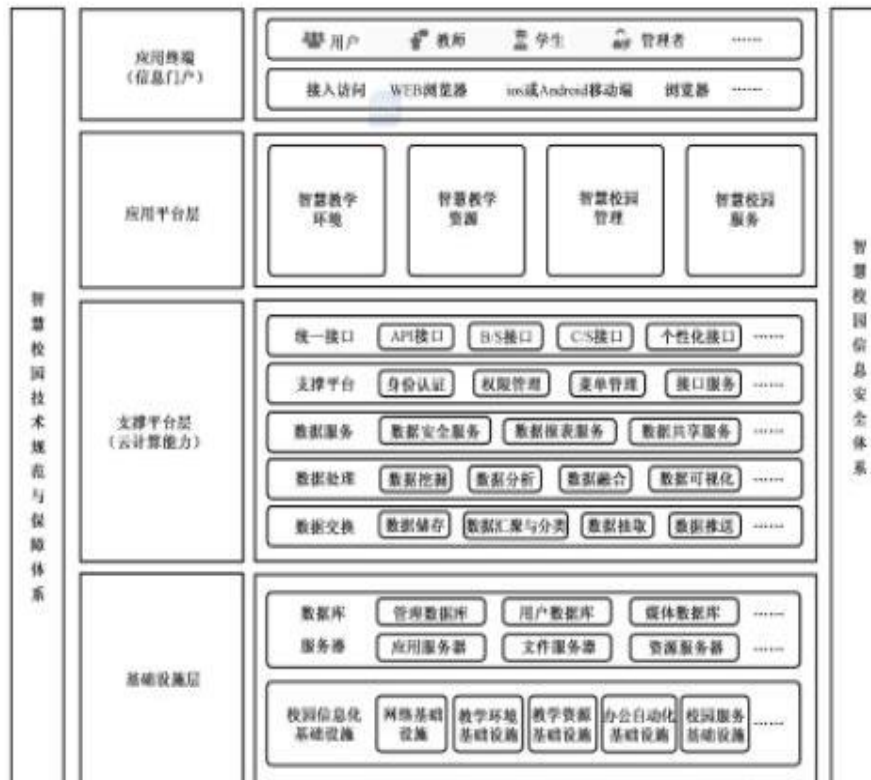
图 1 智慧校园总体架构图
